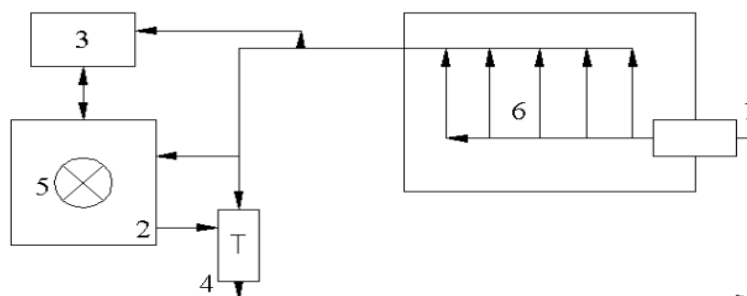
1-rasm. Dvigatelning sovutish tizimi funksional sxemasi.
